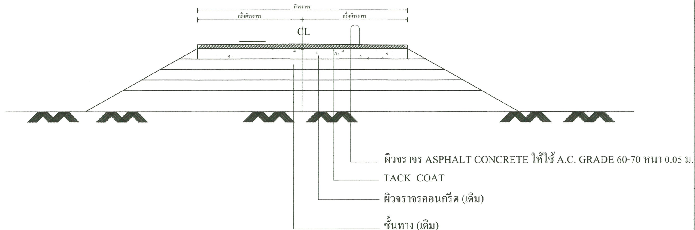
รูปตัดตามขวางงานก่อสร้างถนนแบบ ASPHALT CONCRETE (OVER LAY)
